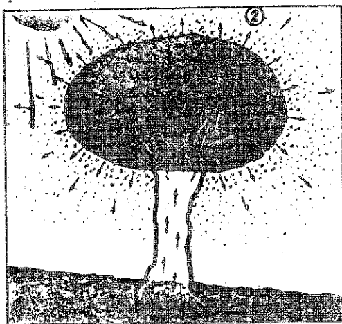
Insolación con árboles
