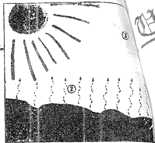
Insolación sin árboles
