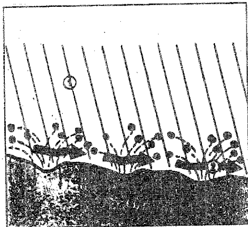
Lluvia sin árboles
