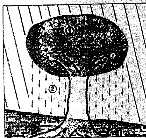
Lluvia con árboles
