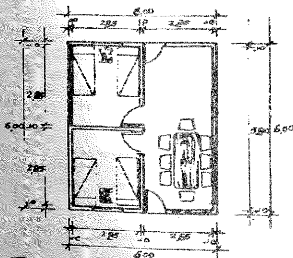
PLANTA 30,00 M 2
